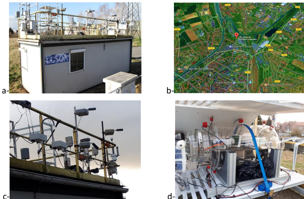
Figure 1 – Station urbaine site de Dorignies IMT Lille Douai. a-shelter avec vue de la plate-forme extérieure, b-positionnement géographique, c-installation des capteurs sur le pourtour de la plateforme, d-chambre d'exposition permettant l'accueil des capteurs non-adaptés en l'état aux conditions extérieures
